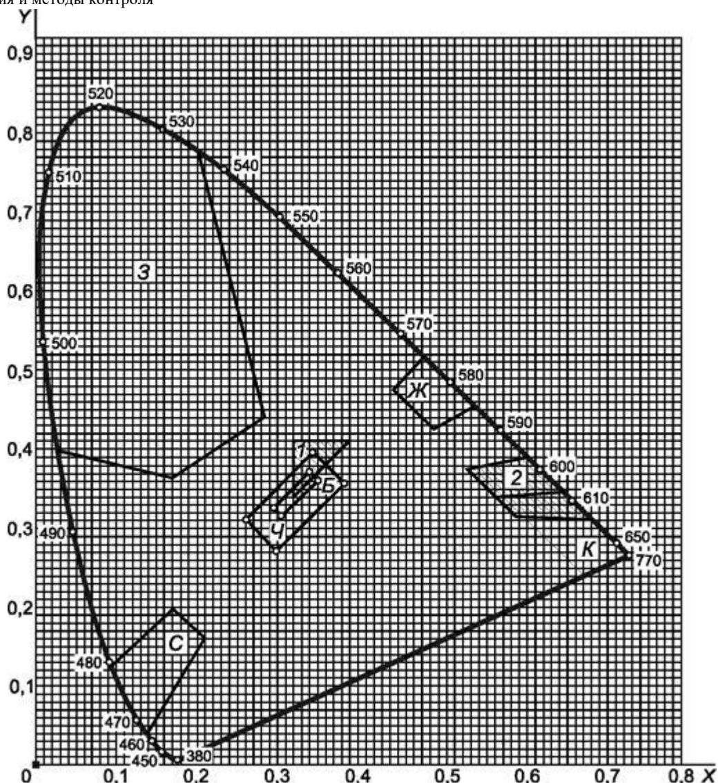
K - область красного цвета; Ж - область желтого цвета; З - область зеленого цвета; С - область синего цвета; Б - область белого цвета; Ч - область черного цвета; 1 - предпочтительная малая область для желтовато-белого фотолюминесцентного цвета; 2 - предпочтительная малая область для красного (красно-оранжевого) фотолюминесцентного цвета
